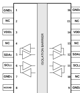
CMT8100 WB SOIC-16
