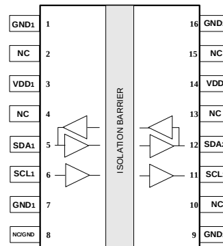
CMT8101 WB SOIC-16
